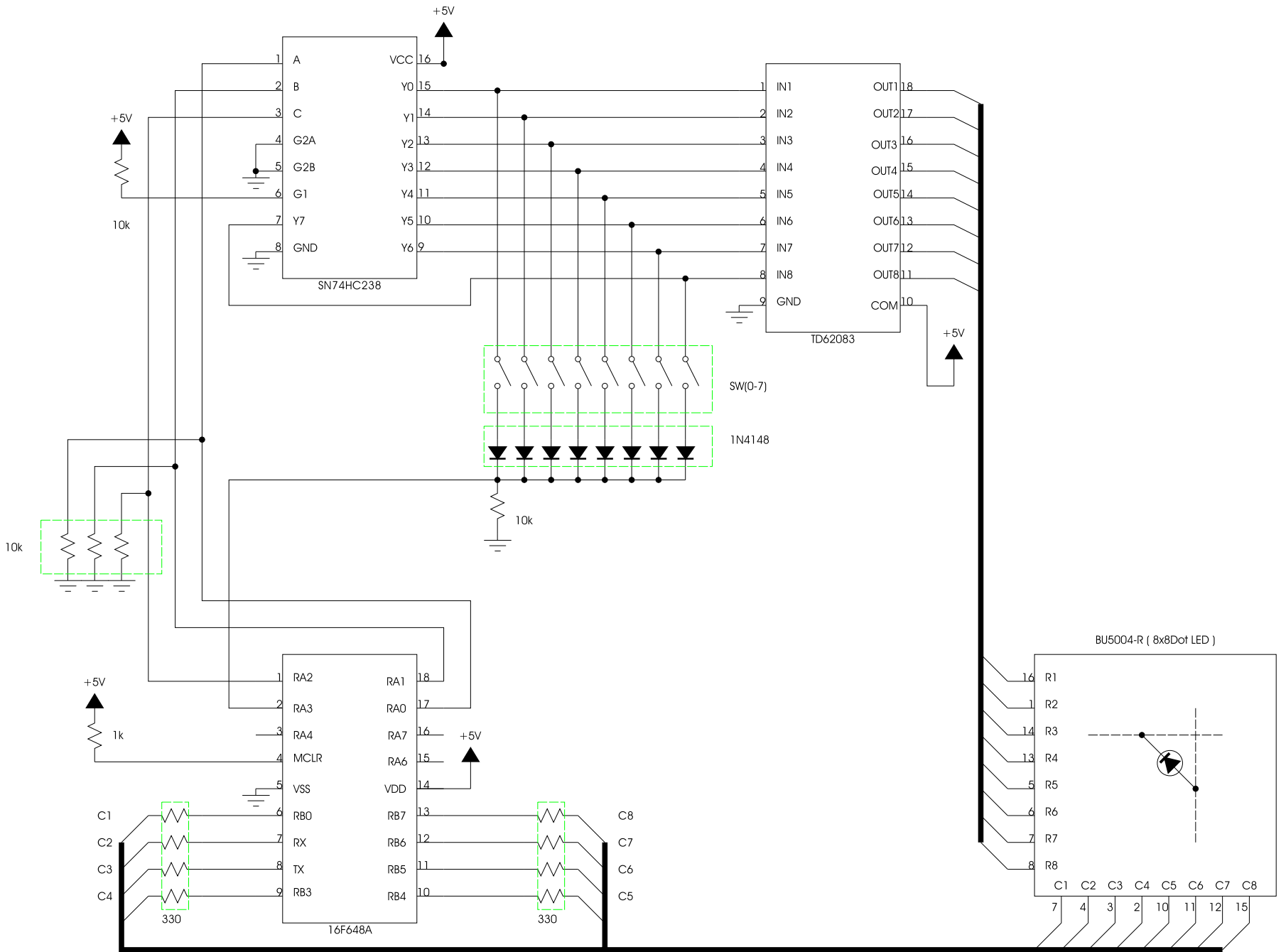
アルゴ算法堂 88ドットLEDドライブ回路 (キー入力付き)
