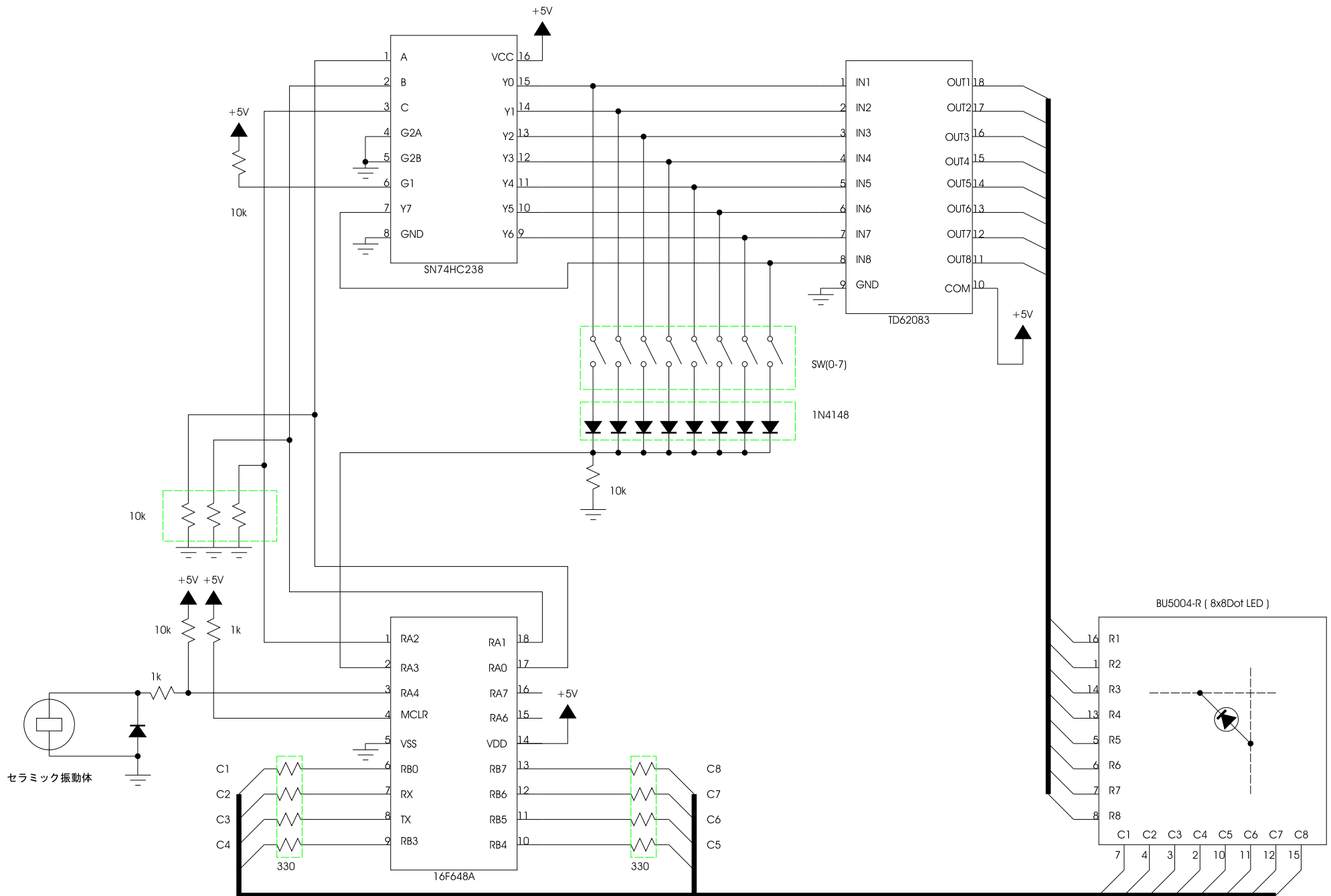
アルゴ算法堂 88ドットLEDドライブ回路 (Key & Buzzer)
